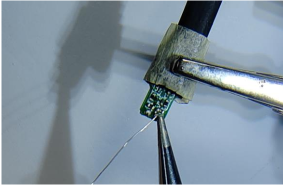
银线焊接
