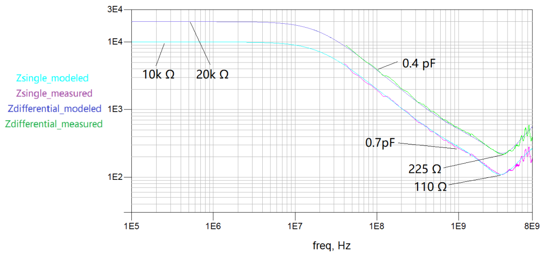
SAP5000D 输入阻抗曲线（焊接 24.9Ω引线电阻）
